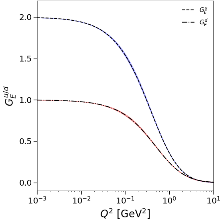
SBS Global Fit
