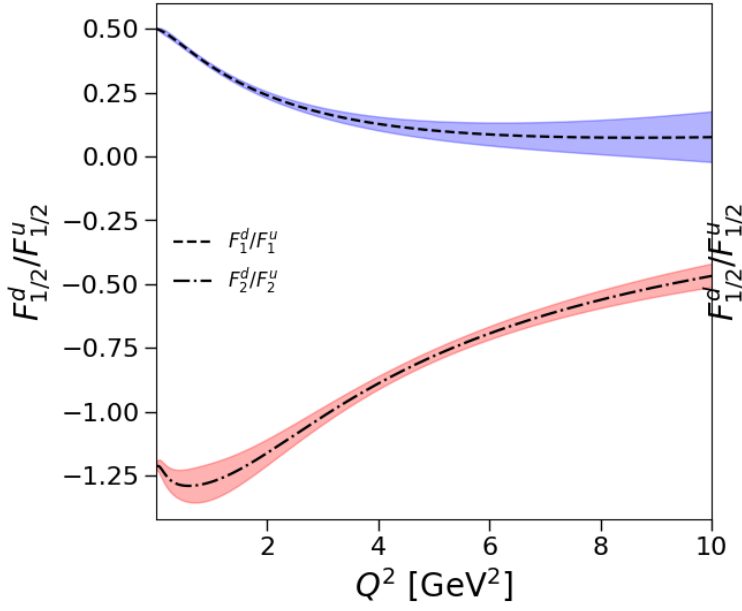
SBS Global Fit
