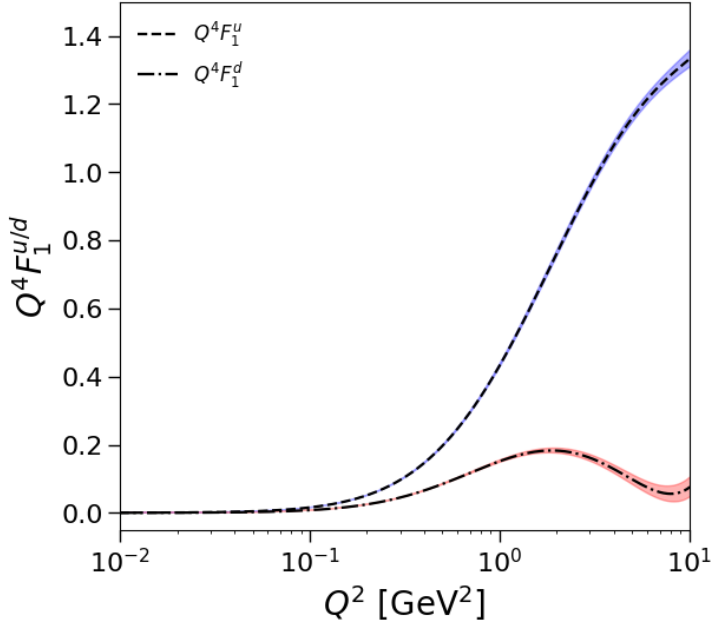
SBS Global Fit
